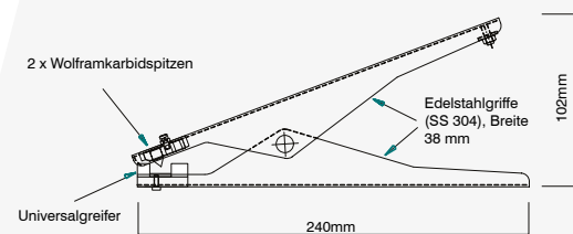
Zweipolige Edelstahlerdungsklammer mit Kontaktspitzen aus Wolframkarbid
