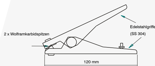
zweipolige Erdungsklammer und zwei Wolframkarbidspitzen
